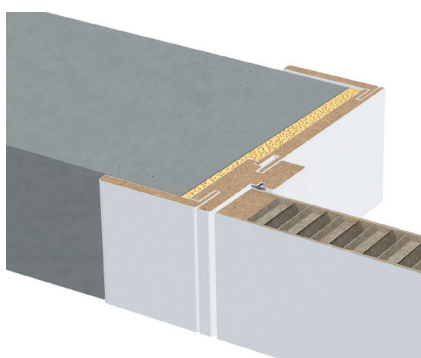
коробка-наличник-полотно лежат в одной плоскости
