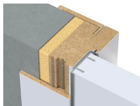
полотно и наличник лежат в одной плоскости, наличник перекрывает часть коробки, что уменьшает количество стыков
