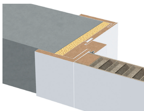
полотно и наличник лежат в одной плоскости, наличник перекрывает часть коробки, что уменьшает количество стыков
